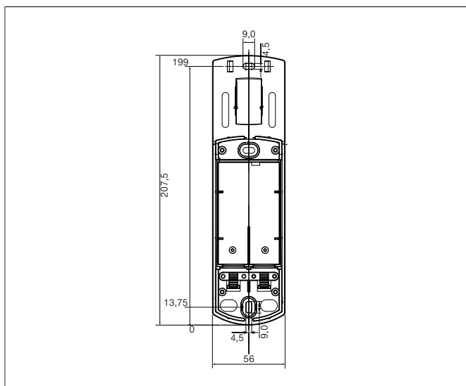
Abb. 2: Abmessungen
