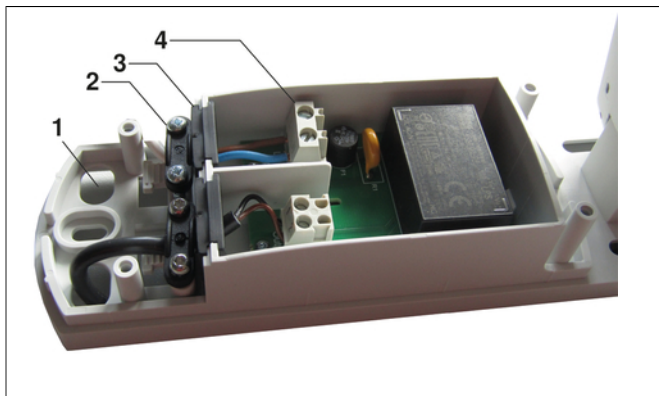
Abb. 7: Anschluss der Wetterstation
